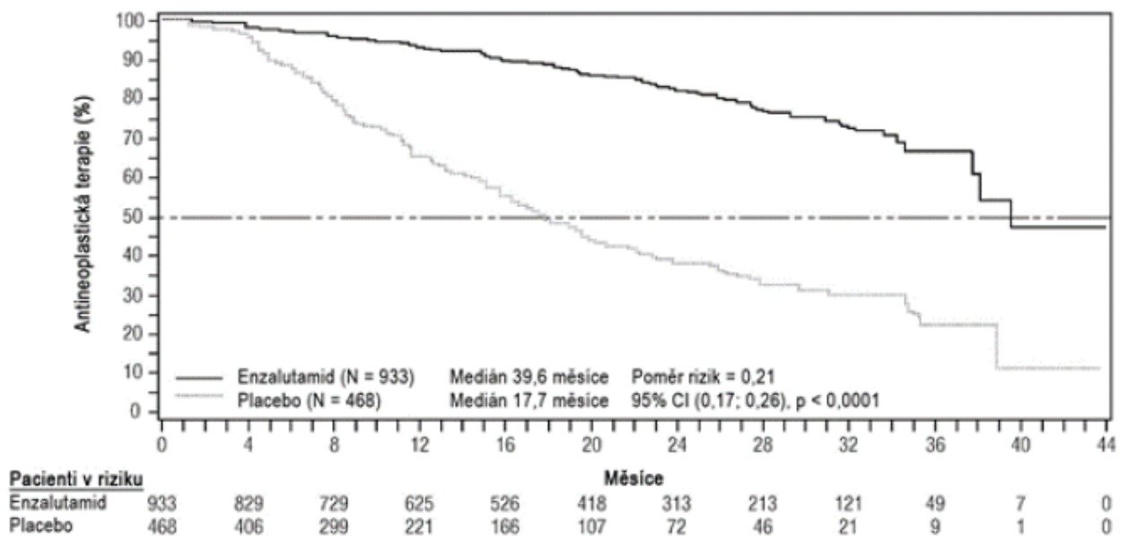
Obrázek 7: Kaplanovy-Meierovy křivky doby do prvního užití nové cytostatické terapie ve studii PROSPER (analýza intent-to-treat)
