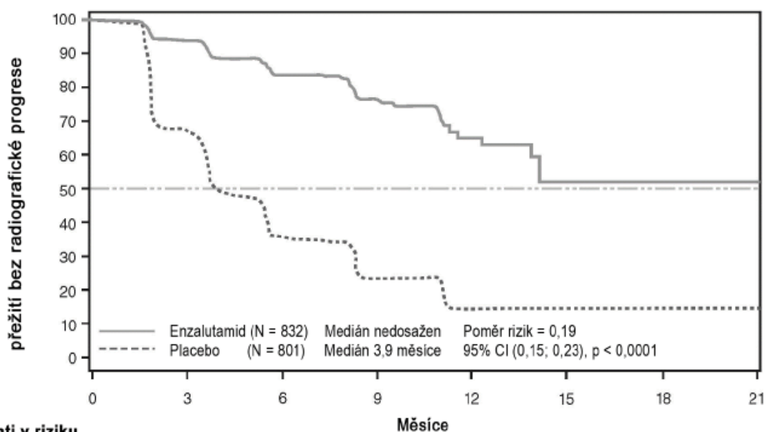
Obrázek 11: Kaplanovy-Meierovy křivky přežití bez radiografické progresie ve studii PREVAIL (analýza intent-to-treat)
