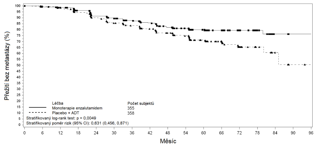
Obrázek 2: Kaplanovy-Meierovy křivky MFS v léčebných ramenech enzalutamid v monoterapii vs. placebo s ADT ve studii EMBARK (analýza intent-to-treat)
